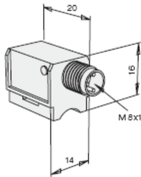
电磁传感器
