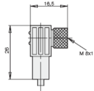
直角插头连接电线
